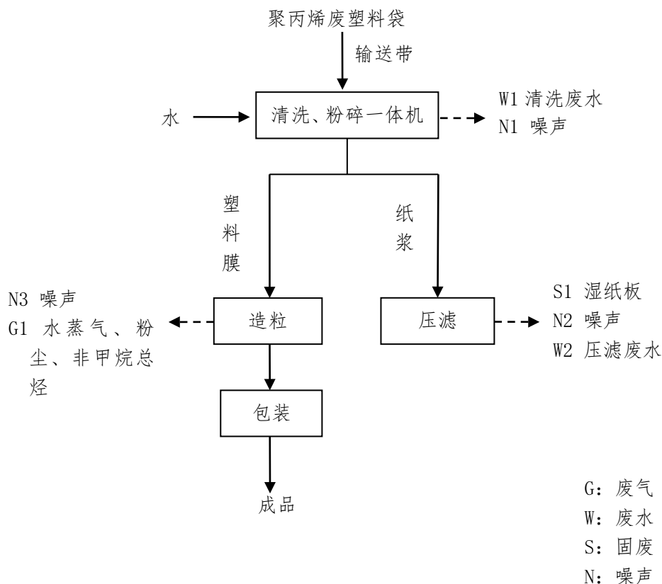
图 2.4-1 生产工艺流程图
